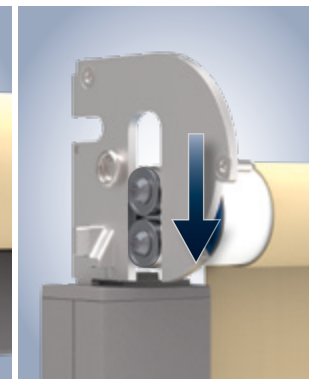
Tuchwelle abgewickelt
