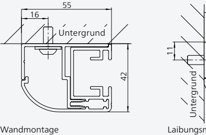
Führungsschiene, rund
