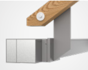
Dachsparrenmontage
